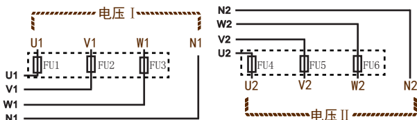
图一 电压信号测量接线方式
